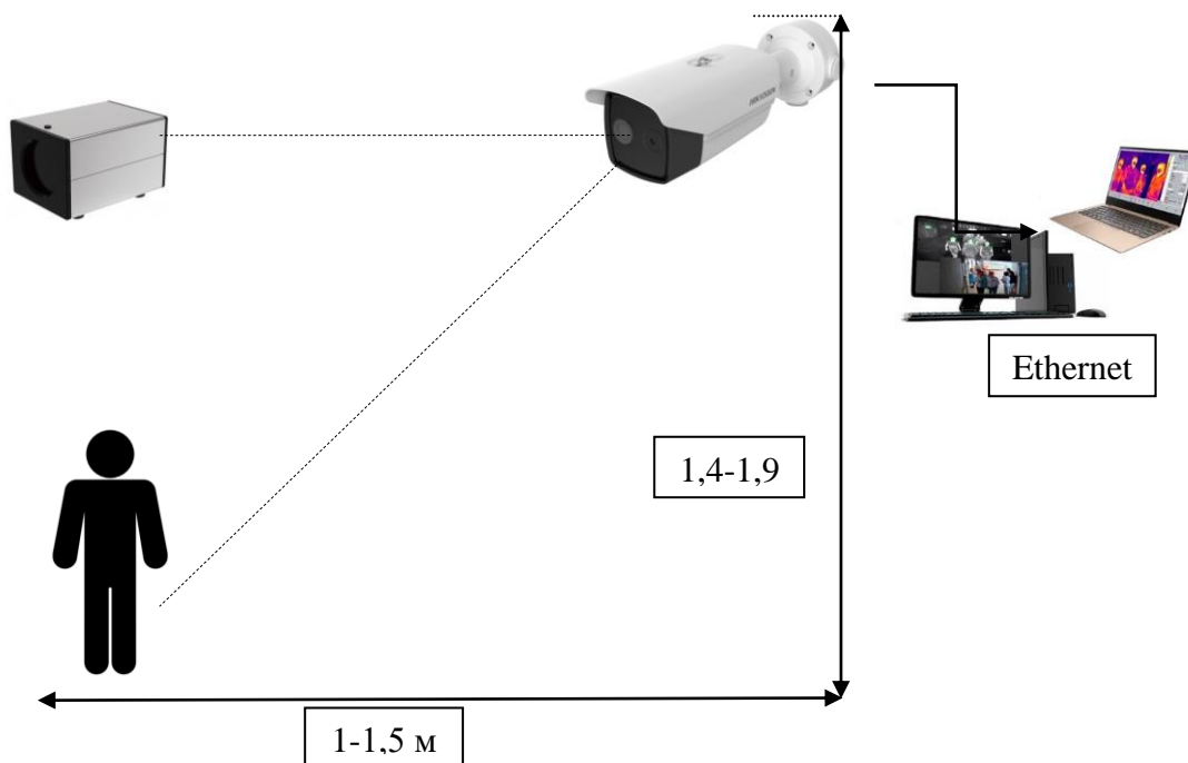
Рисунок 4 – Структурная схема системы
